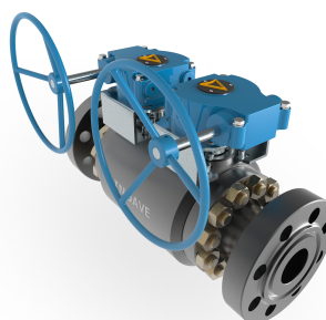
Válvula doble integral (Double Block & Bleed).
