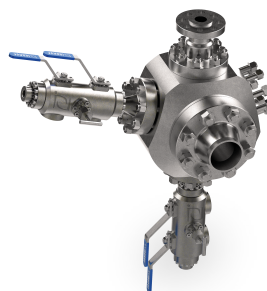
Cubo de conexión API6A.
